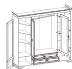
024 Шкаф S320-SZF6D2S 227/225/62,5 шир./выс./глуб.
